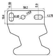
CSD-G50 CGF50 安装架 Mounting bracket
