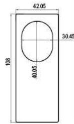
CSD-M30-L M30-L 安装架 Mounting bracket
