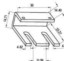
CSD-F30 30x30 安装架 Mounting bracket
